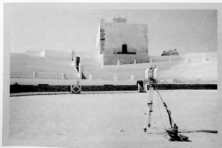
Láser escáner en el Castillo de Barcarrota
